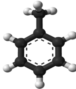
تولوئن
