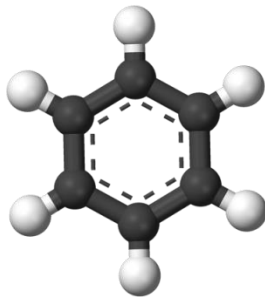
بنزن
