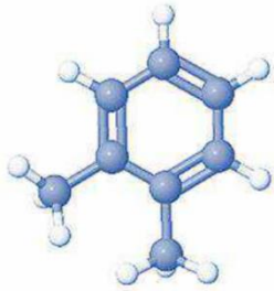
ارتوزایلین
